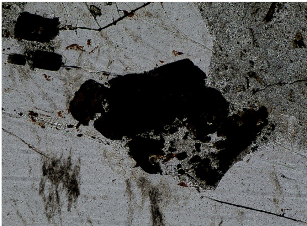
Abb. 8: Unter einfach polarisiertem Licht ist eine hypidiomorph ausgebildete Erzphase zu beobachten, die aus Hämatit bestehen dürfte, was im Dunkelfeld durch die leicht rötliche Färbung erklärt wird.
