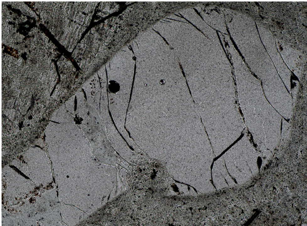
Abb. 4: Abgebildet ist ein Quarzindividuum, das sowohl gerade Kristallflächen, die im Übergang zueinander gerundet sind, als auch tief „eingefressene“ Resorptionsbuchten erkennen lässt (s. weißer Pfeil im Dunkelfeld).
