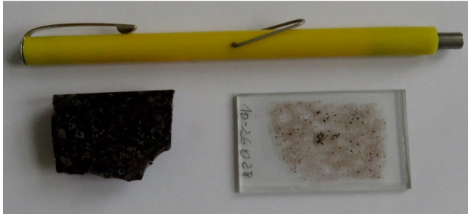
Abb. 2: Dünnschliff der zu untersuchenden Gesteinsprobe 10-26028. (Maßstab: 5 Cent Münze, Querschnitt = 2,0 cm)
