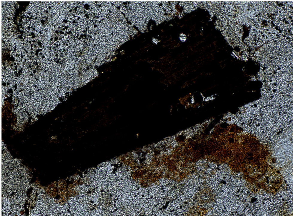
Abb. 7: Unter einfach polarisiertem Licht ist eine Verwachsung aus erzreichen Bereichen (schwarze Färbung) und alteriertem Biotit-Individuum zu erkennen. Deutlich wird die fast den ganzen Biotit einnehmende Erzphase, die aus Hämatit bestehen dürfte, was aber in der Durchlichtmikroskopie nicht genauer bestimmt werden kann.
