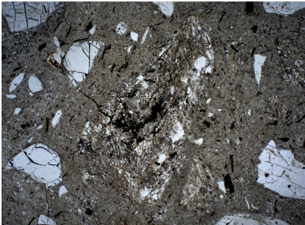
Abb. 6: Der abgebildete Kalifeldspat ist stark sericitisiert und bildet nach dem Karlsbader Gesetz Zwillinge aus. Untere Bildkante 2 mm Durchlicht: oben + Nicols; unten // Nicols
