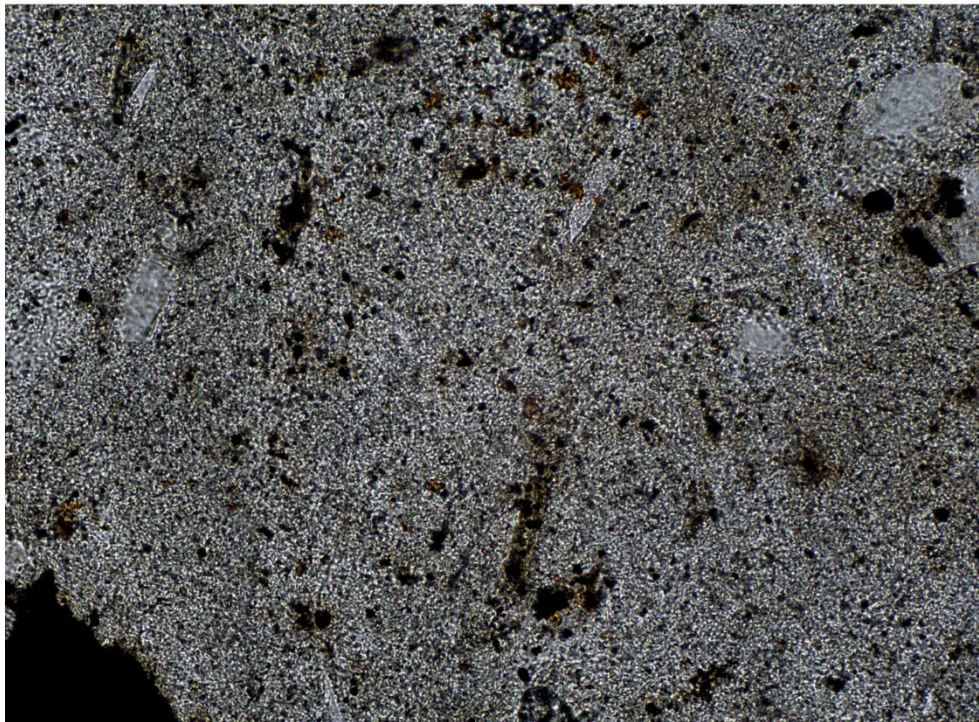
Abb. 9: Die Matrix ist sehr feinkörnig ausgebildet und besteht aus einem feinen Gemenge: Quarz, Plagioklas, Kalifeldspat und Hämatit.
